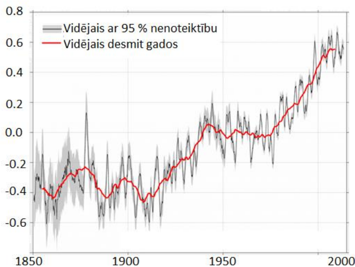
1. Att. Zemes virsmas temperatūra no 1850 gada līdz 2000 gadam[1]
